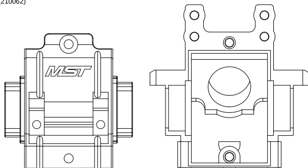
FXX Rear gear box set FXX 後齒箱組 (210062)
