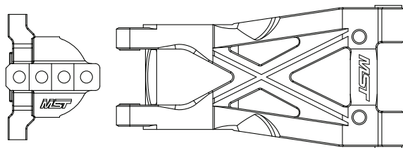
HT Rear lower arm & wheel hub ×2 HT 後下擺臂&輪座 210055
